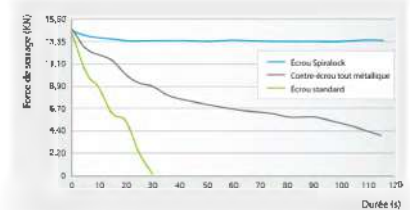
Paramètres du test : Écrous M6 à 20 Hz avec une amplitude de mouvement transversal de 0,6 mm
